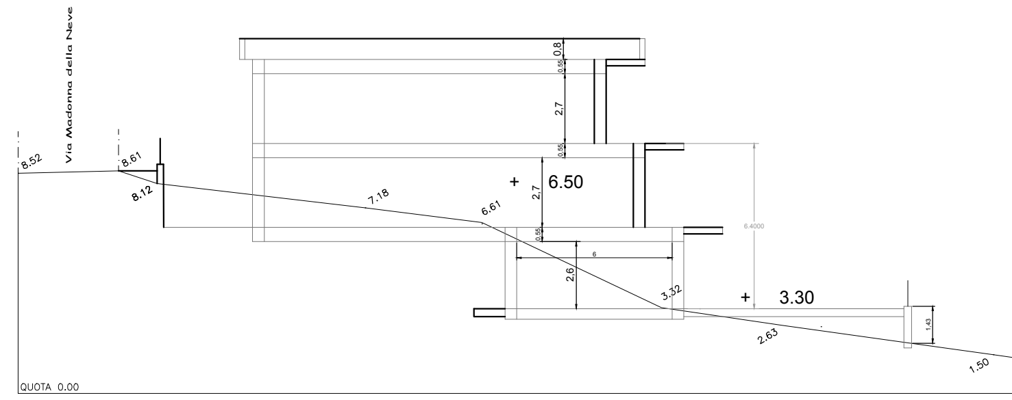
Sezione Schematica A-A
